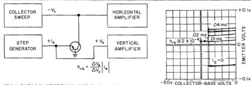
(D) VOLTAGE FEEDBACK RATIO, h_{ie} , h_{rb}
