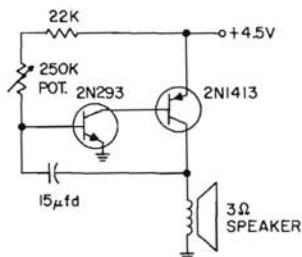
METRONOME
