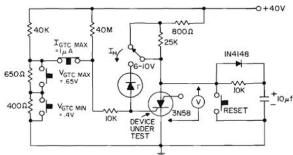
DC PARAMETER TEST SET FOR 3N58
