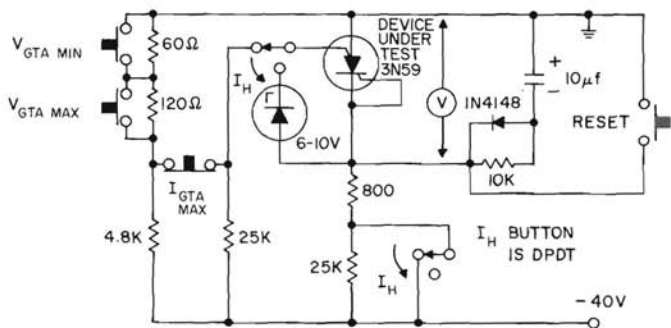
DC PARAMETER TEST SET FOR 3N59
